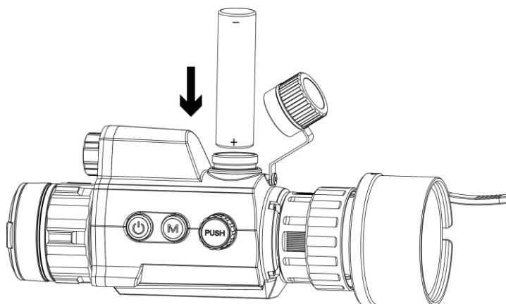
Obrázok 2-4 Inštalácia batérie
