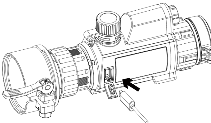
Obrázok 2-1 Káblové pripojenie
