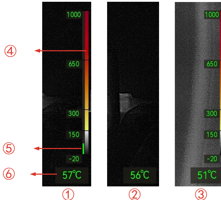
図 4-1 サーマル読み取り
