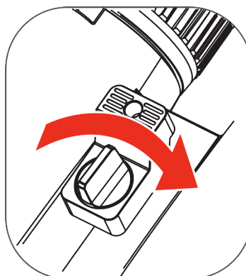
Рис. 2-14 Поворот винта
