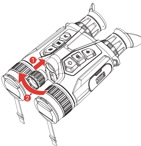
Рис. 2-8 Установка осветителя
