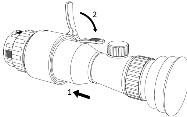
Abbildung 2-3 Tageslichtzielfernrohr montieren
