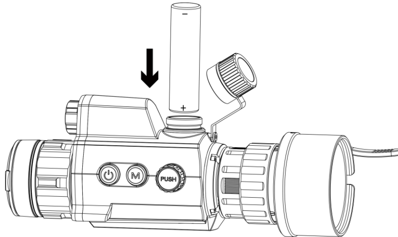
Abbildung 2-5 Akku einlegen
