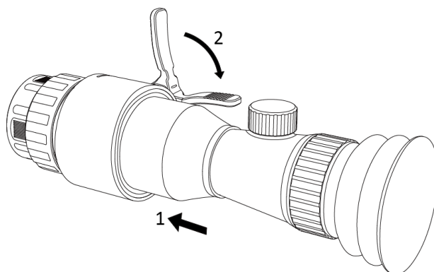
Figur 2-3 Montera dagsljuskikarsikte
