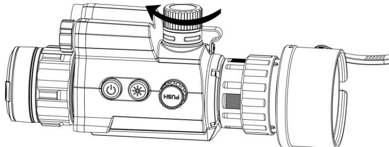
Figur 2-6 Stäng batteriluckan
