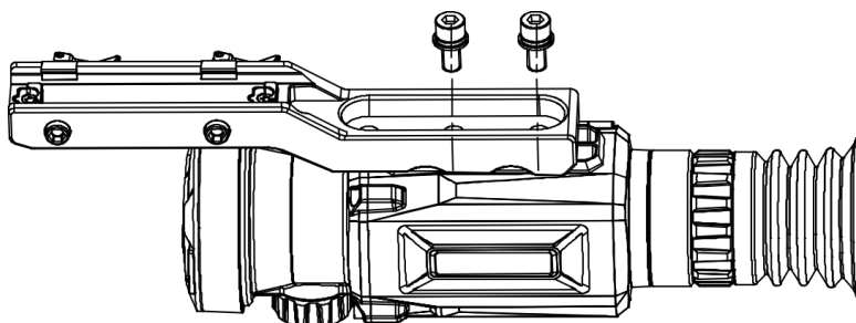
Obrázok 2-5 Vloženie skrutiek
