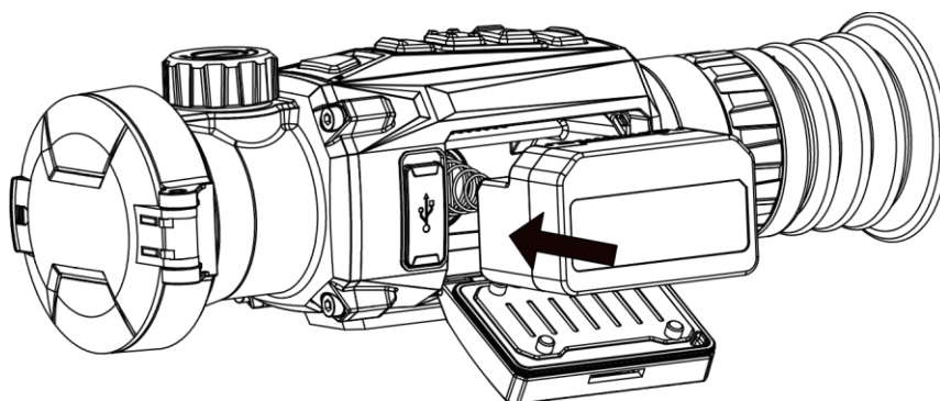
Obrázok 2-3 Vloženie batérie
