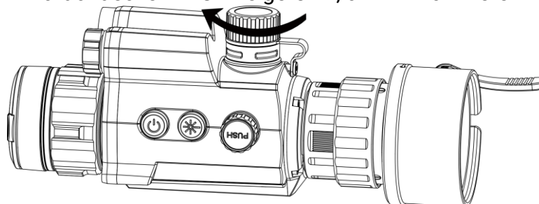
Figure 2-6 Akkufachdeckel schließen
