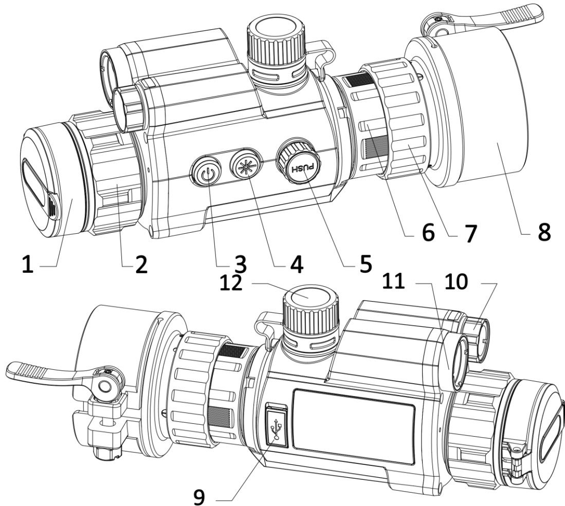
Abbildung 1-1 Aussehen des Geräts
