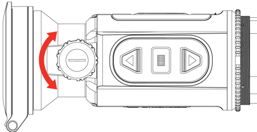
Abbildung 3-1 Fokus einstellen
