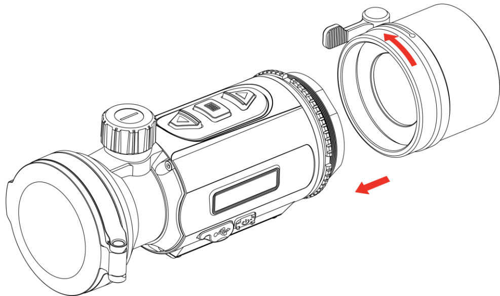
Abbildung 2-6 Adapter montieren
