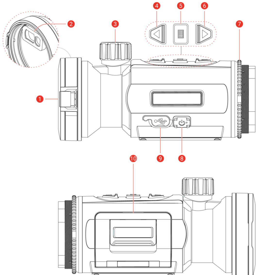
Abbildung 1-1 Aufbau
