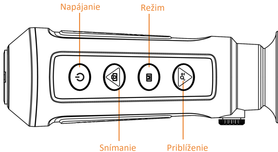
Obrázok 1-1 Tlačidlá na zariadení
