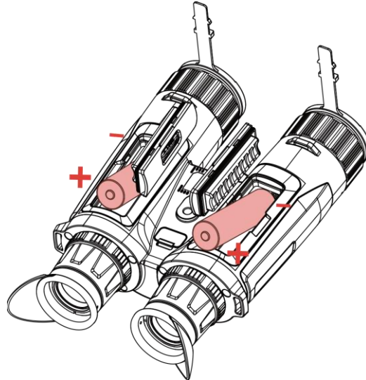
Figure 2-2 Installation de la batterie
