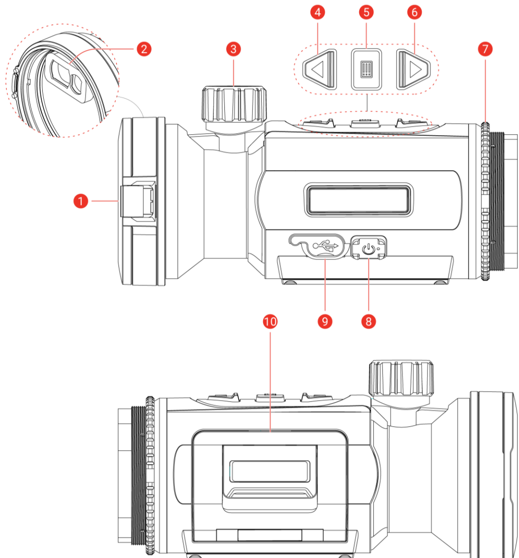
Abbildung 1-1 Aufbau
