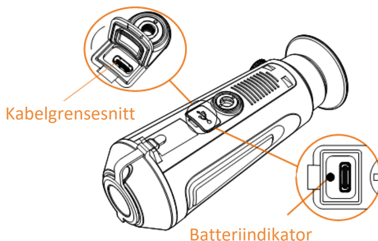
Figur 2-1 Kabelgrensesnitt
