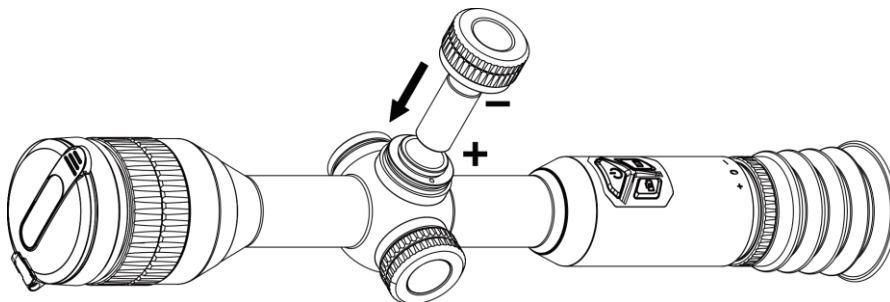
그림 2-3 배터리 설치
