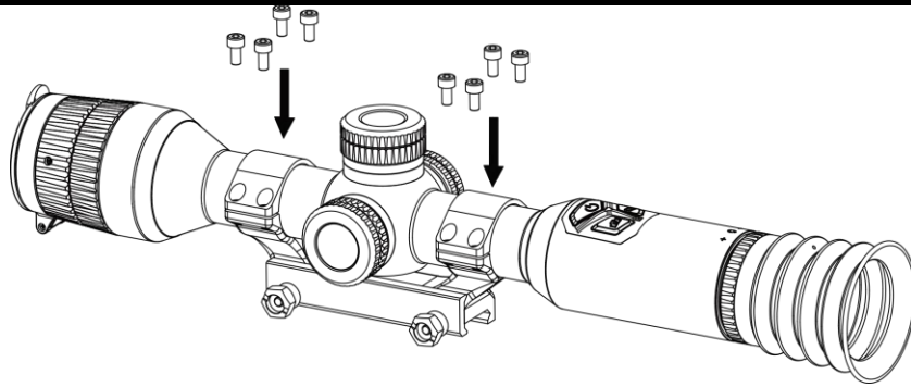
그림 2-7 나사 조이기
