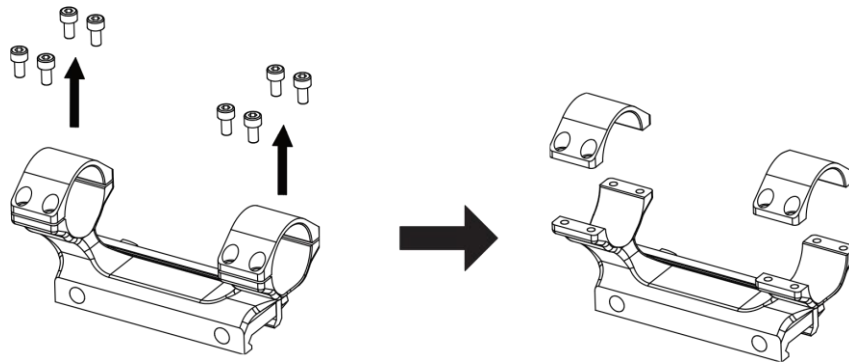
그림 2-5 링 상단 나사 풀기
