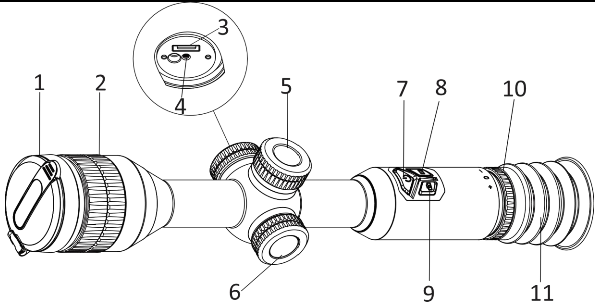
그림 1-1 버튼 및 구성요소
