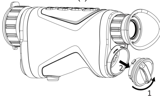
Abbildung 2-1 Abdeckung lösen
