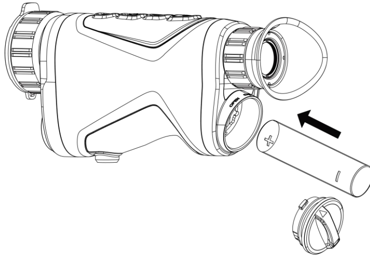
Abbildung 2-2 Akku installieren
