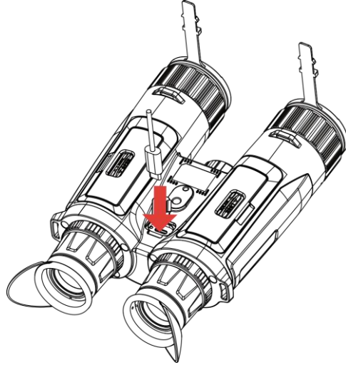
그림 2-4 케이블 연결
