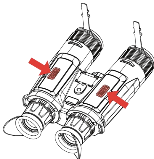
그림 2-1 커버 열기
