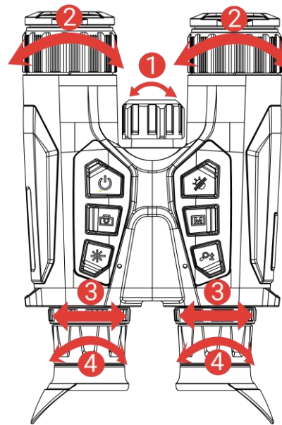
그림 3-1 장비 조정
