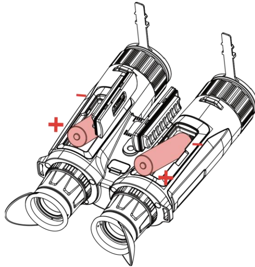
그림 2-2 배터리 설치하기
