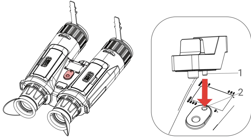
그림 2-8 칼럼 삽입
