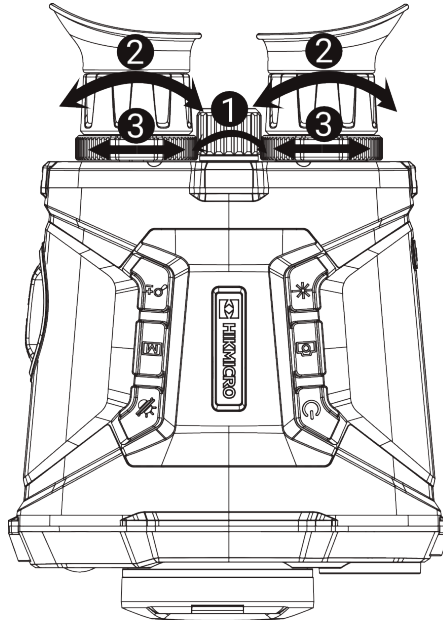
Abbildung 3-1 Gerät anpassen
