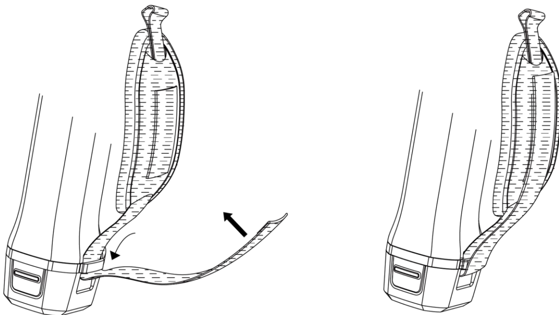
Figure 2-4 Fixation de la partie inférieure de la dragonne
