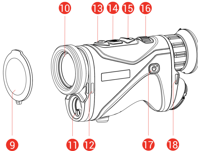
Abbildung 1-1 Aufbau
