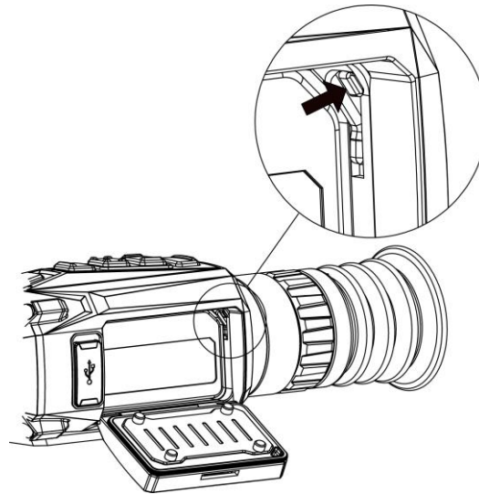
Figura 2-2 Quitar el pestillo de la pila
