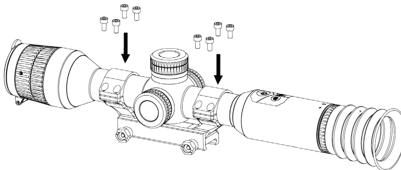
Obrázek 2-7 Utažení šroubů
