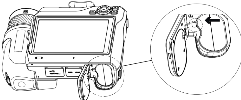
그림 2-3 배터리 해제
