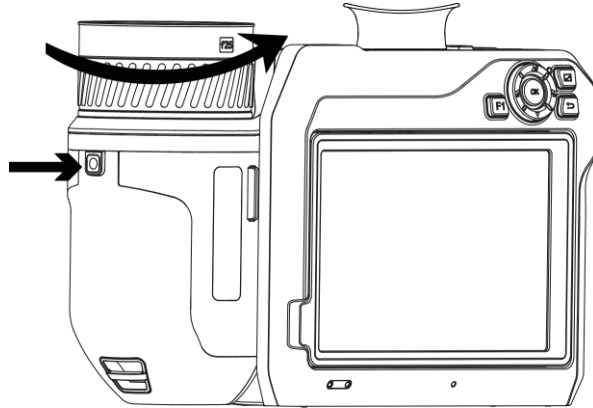
그림 2-6 렌즈 분리
