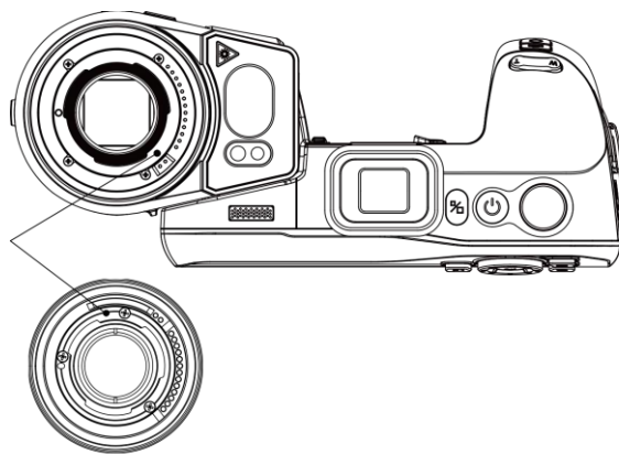
그림 2-8 흰색 표시 정렬
