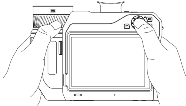
그림 2-18 버튼 제어
