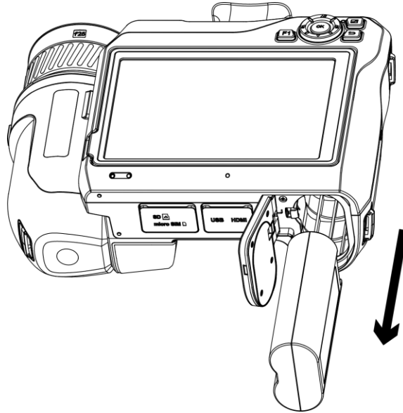
그림 2-4 배터리 제거
