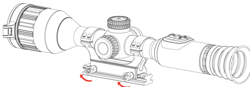
Obrázok 2-9 Uťahnutie skrutiek
