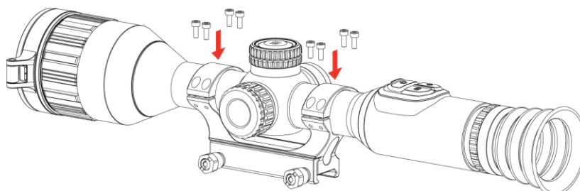
Obrázok 2-7 Uťahnutie skrutiek
