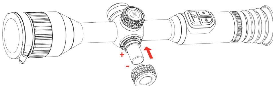
Obrázok 2-3 Vloženie batérie
