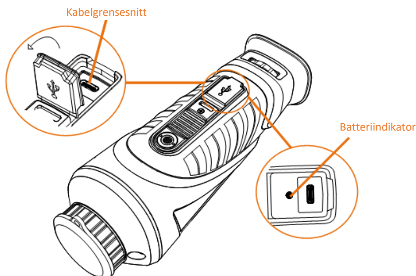
Figur 2-1 Kabelgrensesnitt
