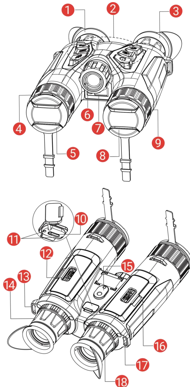
Figur 1-1 Udseende
