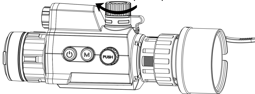
Figura 2-5 Cerrar la tapa de la batería
