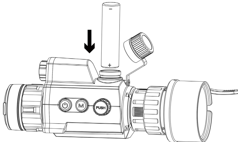
Figura 2-4 Instalar la batería
