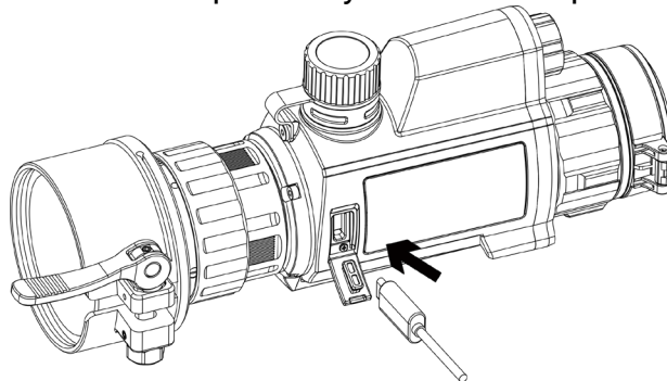
Figura 2-1 Conexión del cable
