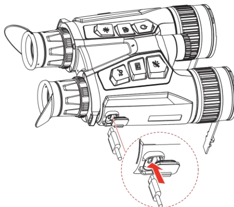
Obrázok 2-5 Nabíjanie zariadenia
