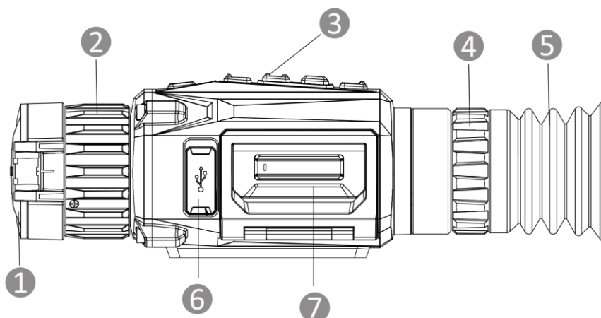
Figur 1-1 Udseende I
