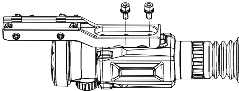
Figur 2-5 Sæt skruer i
