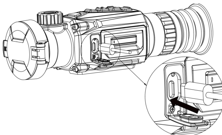
Figur 2-1 Kabeltilslutning
