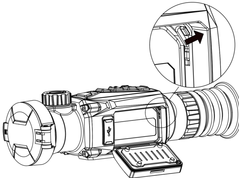
Figur 2-3 Udløs batterilåsen
