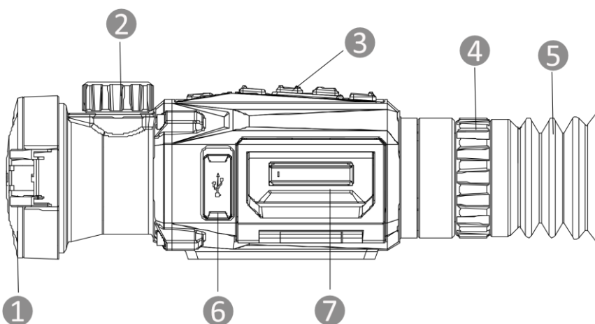
Figur 1-2 Udseende II
