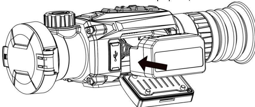
Figur 2-4 Sæt batteriet i
