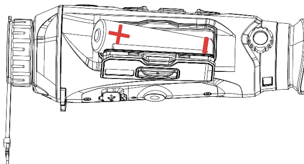
Figura 2-2 Inserimento della batteria
