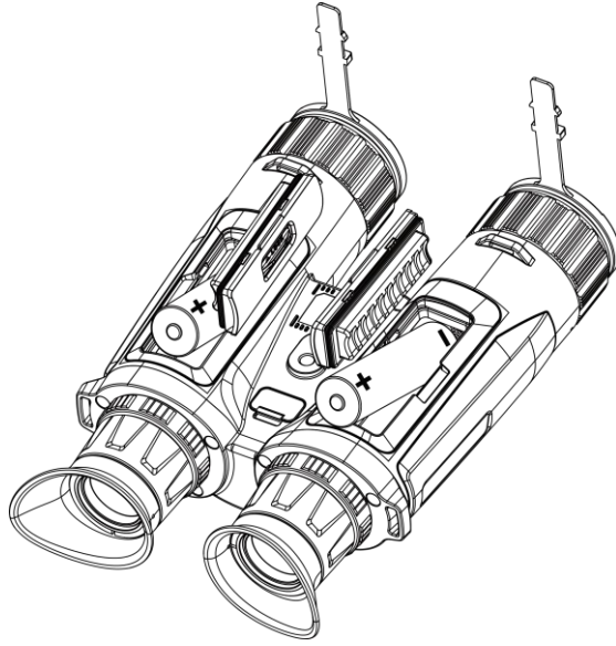
그림 2-2 배터리 설치하기
