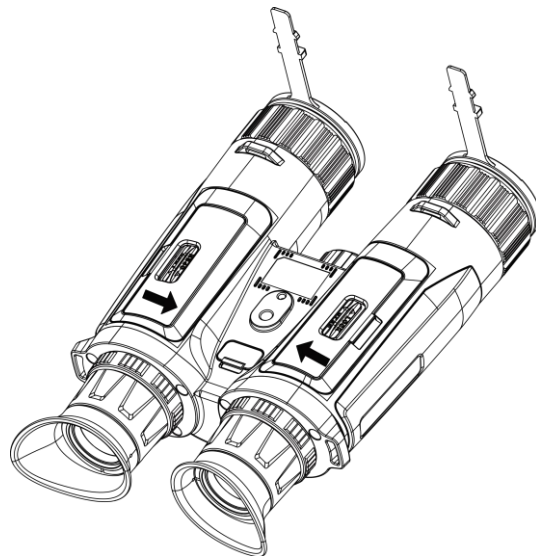
그림 2-1 커버 열기
