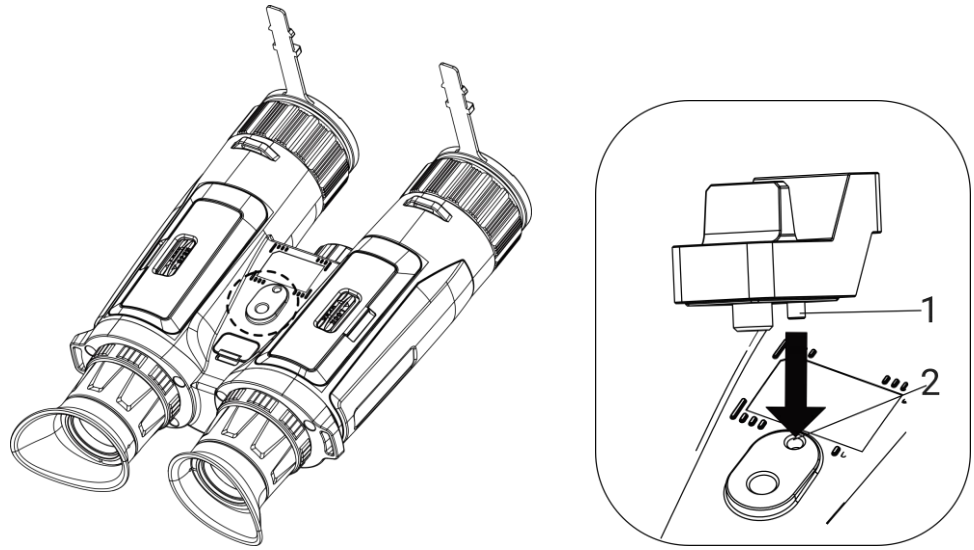
그림 2-8 칼럼 삽입
