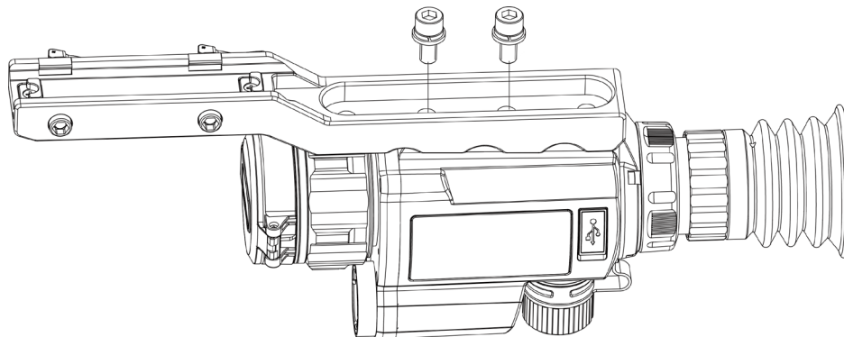
Figur 2-6 Isæt skruer
