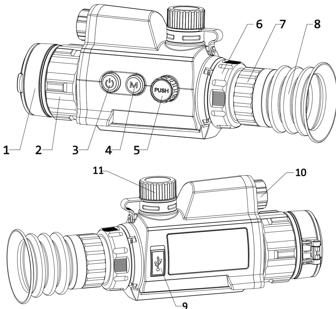
Figur 1-1 Enhedens udseende
