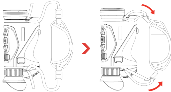
Figura 2-8 Fissaggio della cinghia
