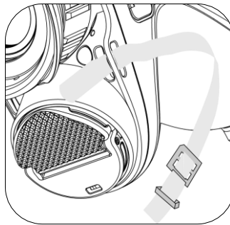
Figura 2-5 Inserimento della tracolla nel punto di attacco
