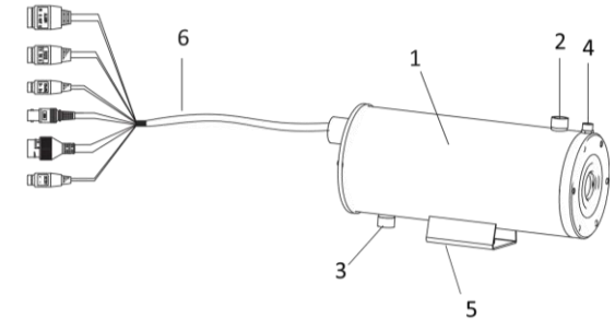
Abbildung 2-1 Aufbau
