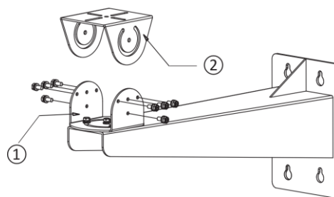
Figur 3-3 Afmontering af PT-beslag
