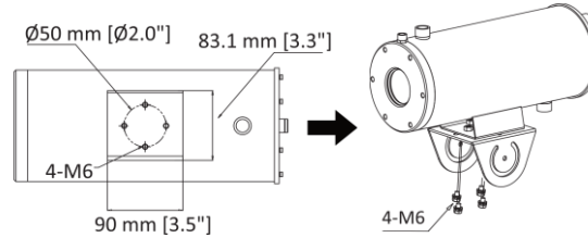
圖 3-6 隨攝影機安裝 PT 接頭頂部
