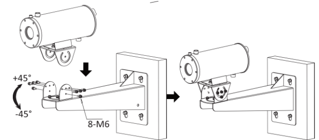
圖 3-7 調整傾斜角度
