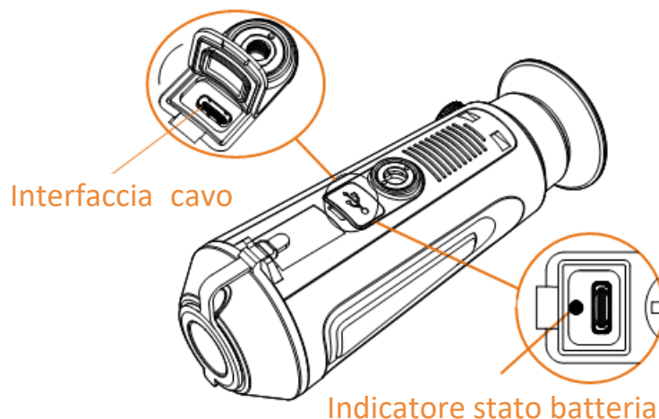
Figura 2-1 Interfaccia cavo
