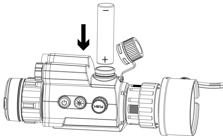
Abbildung 2-4 Akku einsetzen
