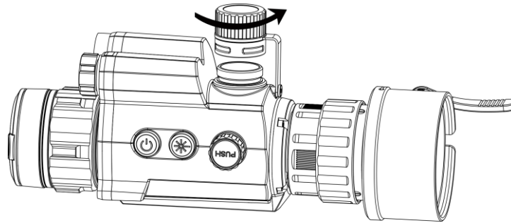
Abbildung 2-3 Batterieabdeckung öffnen
