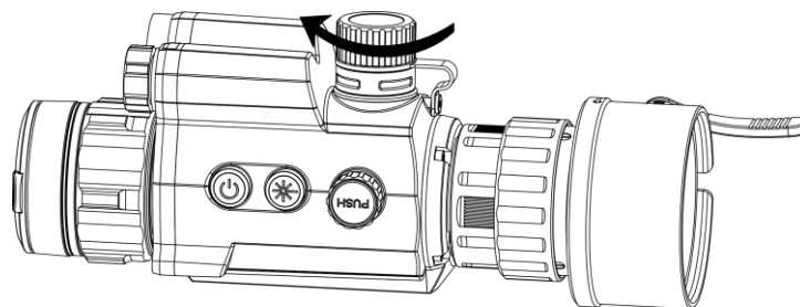
Abbildung 2-5 Batterieabdeckung schließen
