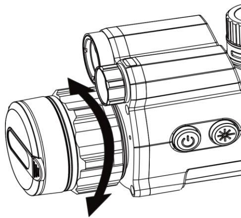
Abbildung 3-1 Fokus einstellen
