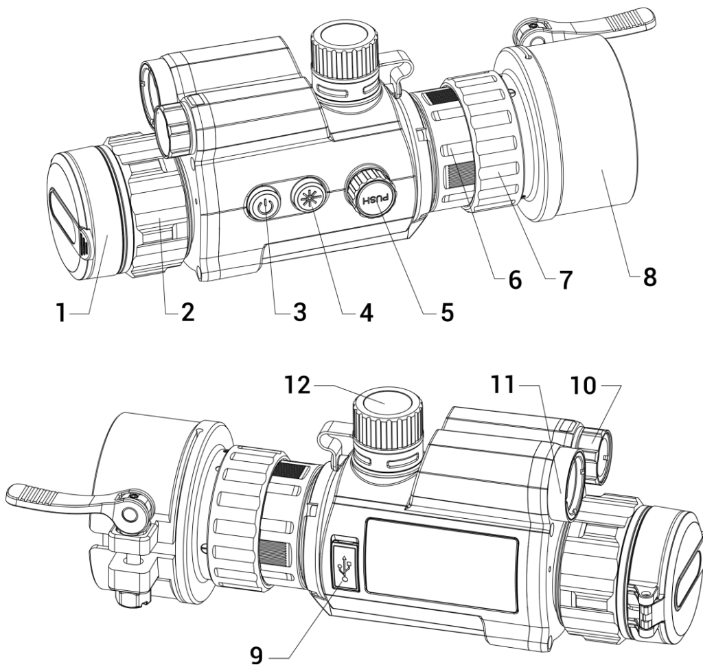
Abbildung 1-1 Gerät Erscheinungsbild
