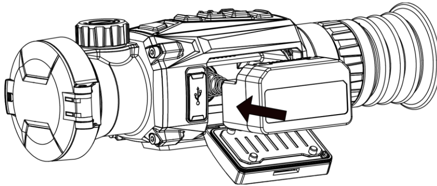
Figure 2-4 Insérer la batterie
