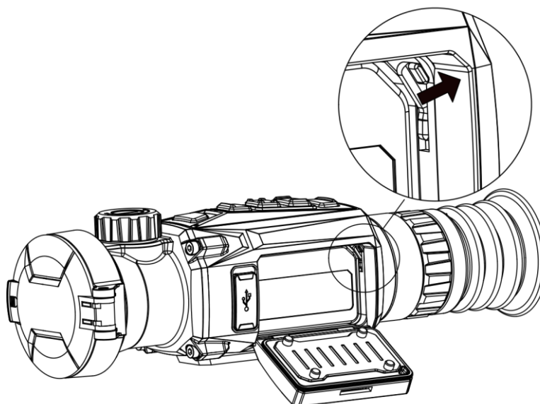
Figure 2-3 Déverrouiller le loquet de la batterie
