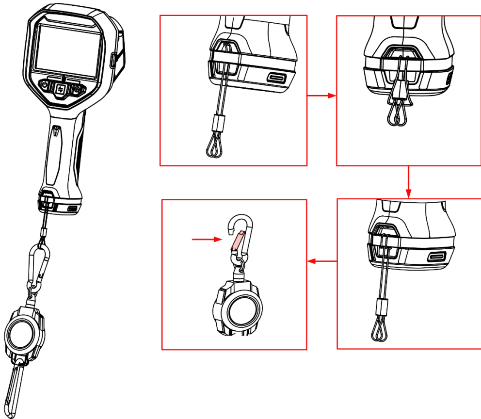
그림 1-5 렌야드 설치
