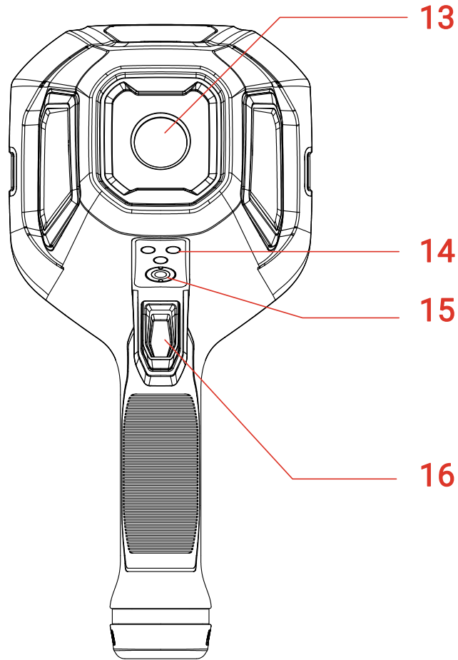
그림 1-2 모양(배면도)
