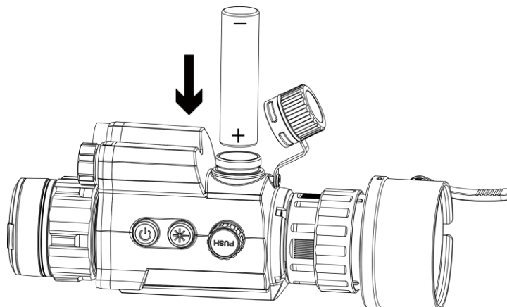
Obrázek 2-4 Vložení baterií
