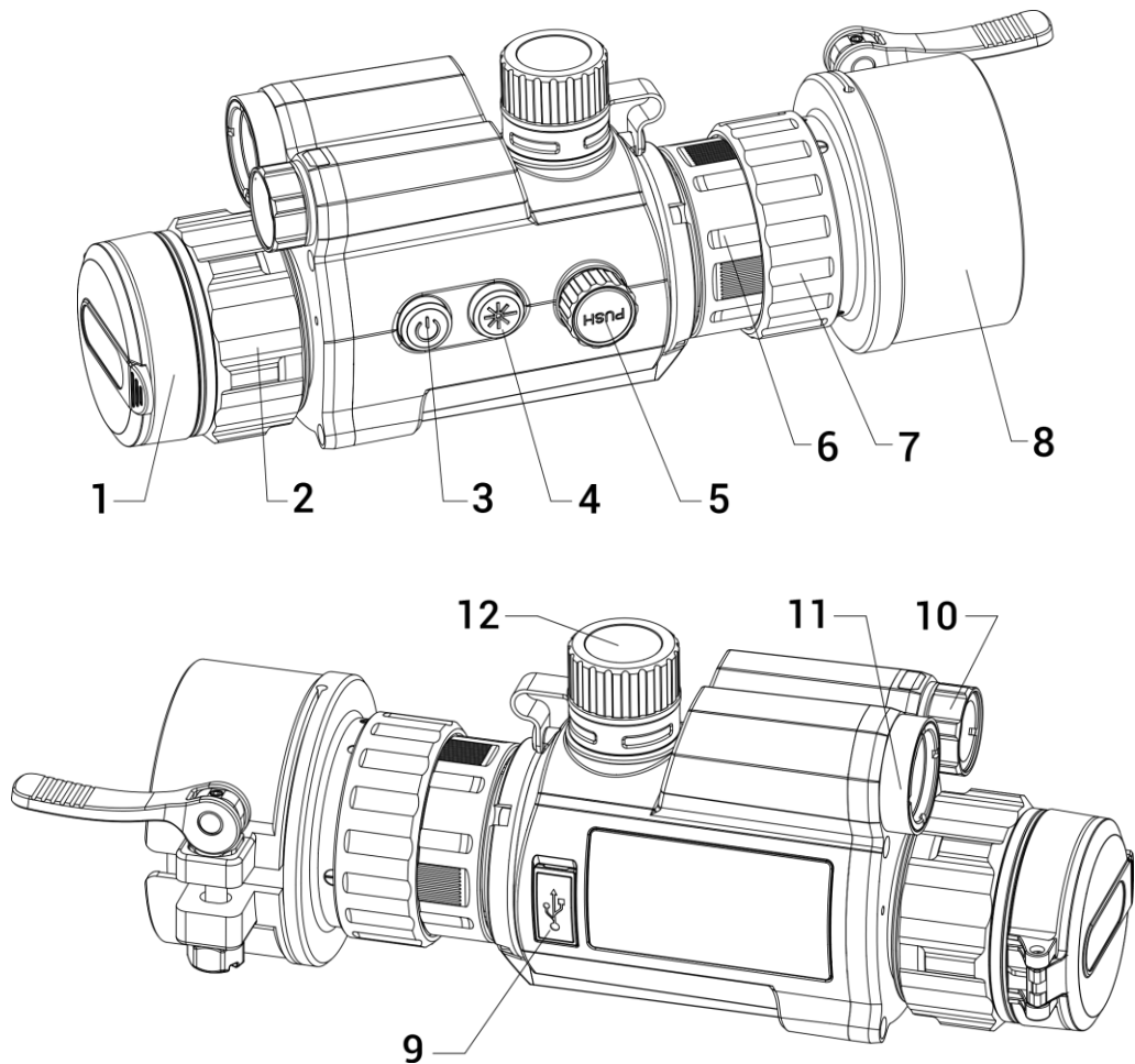
Obrázek 1-1 Vzhled zařízení
