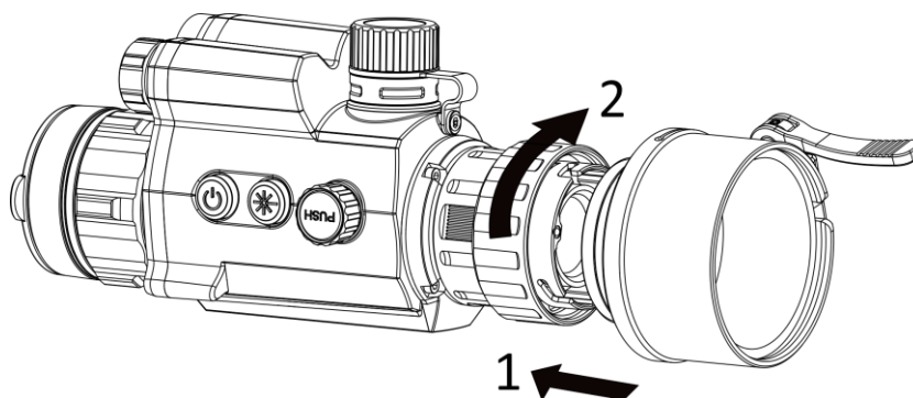
Obrázek 2-2 Montáž adaptéru
