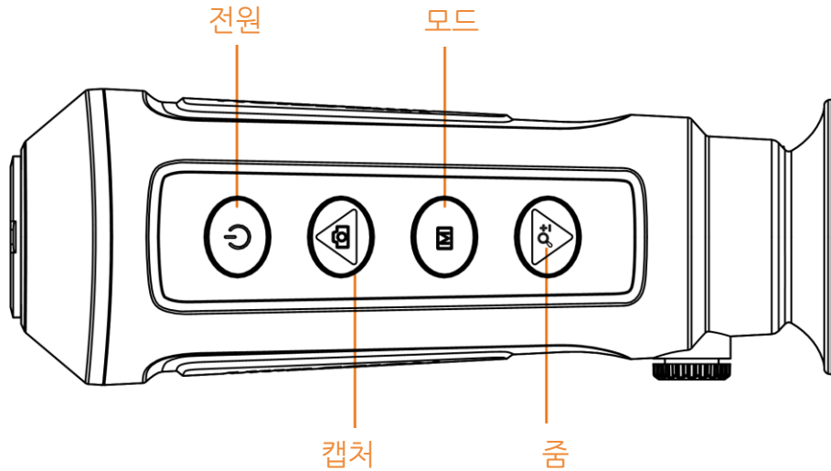
그림 1-1 장비의 버튼
