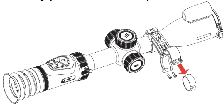
Figur 2-12 Fjern avstandsstykket
