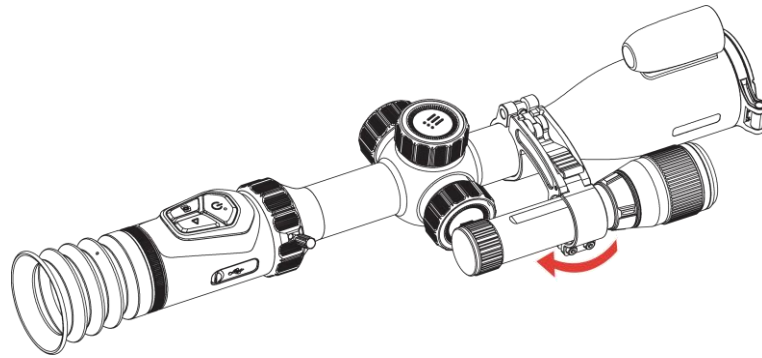
Figur 2-15 Feste IR-lampen
