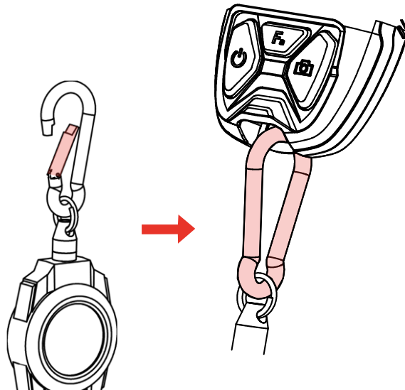
그림 1-5 랜야드 설치
