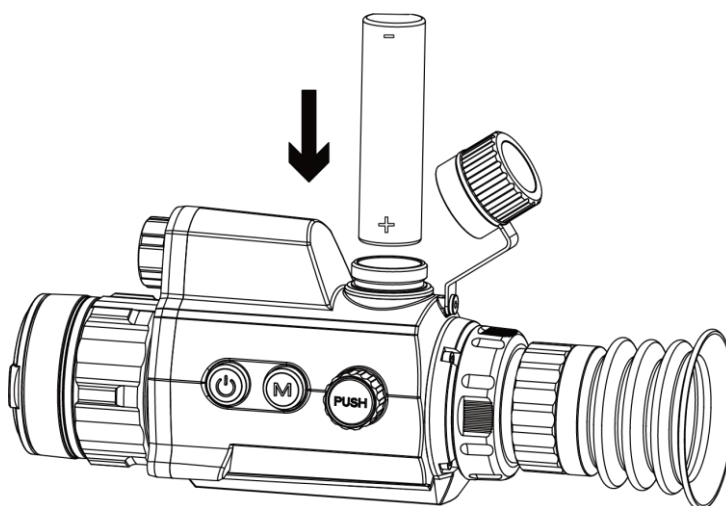
Obrázek 2-3 Vložení baterií
