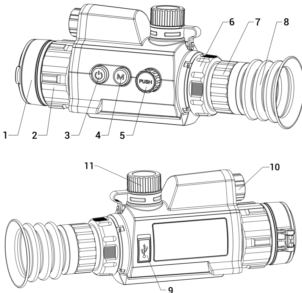
Obrázek 1-1 Vzhled zařízení
