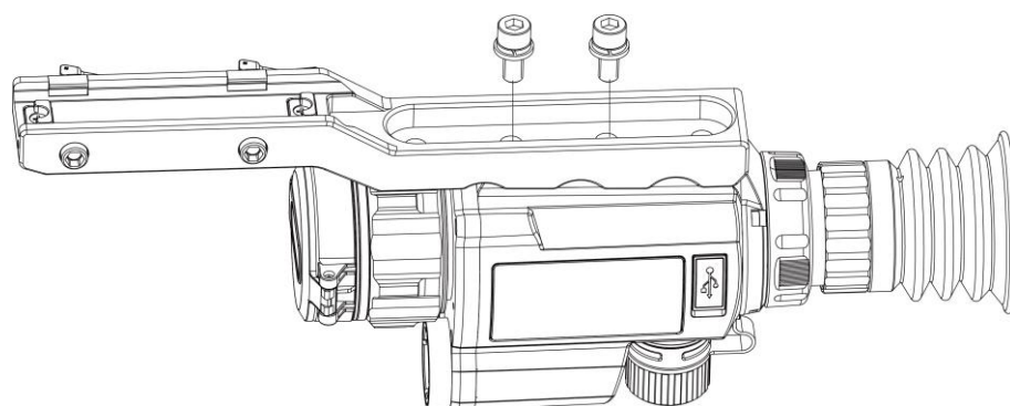
Obrázek 2-6 Namontujte šrouby
