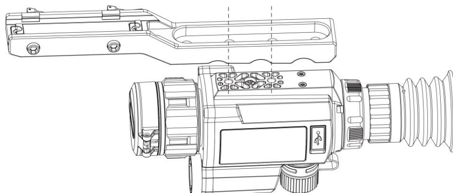
Obrázek 2-5 Zarovnejte instalační otvory
