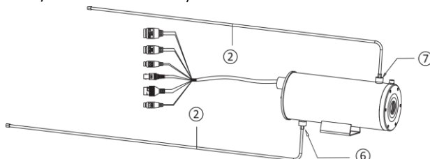
3-10 ábra Vízhűtés csövének csatlakoztatása
