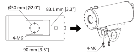
Rysunek 3-6 Mocowanie górnej części uchwyty uchylnego do kamery
