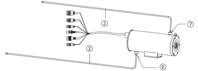
그림 3-10 수랭식 파이프 연결
