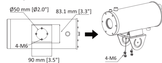
Afbeelding 3-6 De bovenkant van het PT-verbingsstuk installeren op de camera
