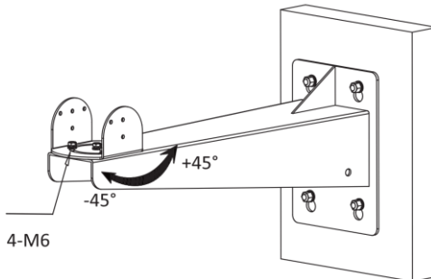
Abbildung 3-5 Schwenkwinkel anpassen
