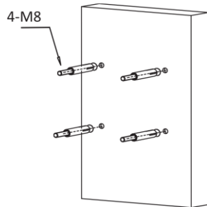
図 3-1 壁にドリルで穴を開ける
