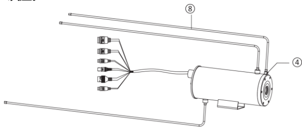
圖 3-11 除塵安裝
