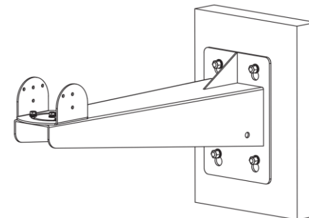
Obrázek 3-4 Instalace držáku
