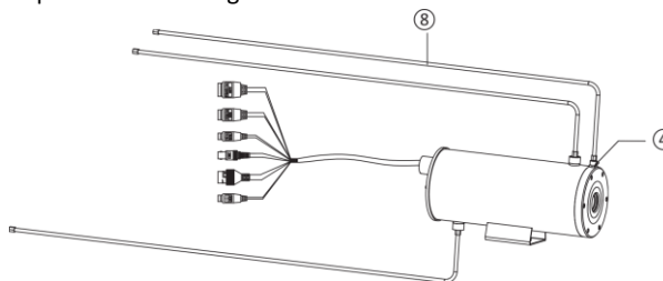
3-11 ábra Portalanítás felszerelése
