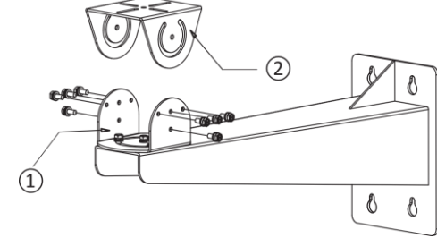
Şekil 3-3 PT Bağlantısını Sökün
