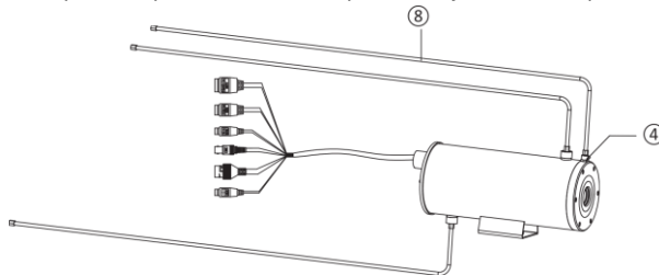
Figura 3-11 Instalação de despoejamento
