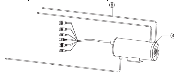
Obrázok 3-11 Inštalácia odprašovania
