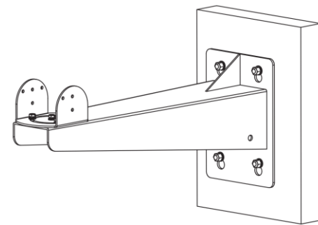
圖 3-4 安裝支架
