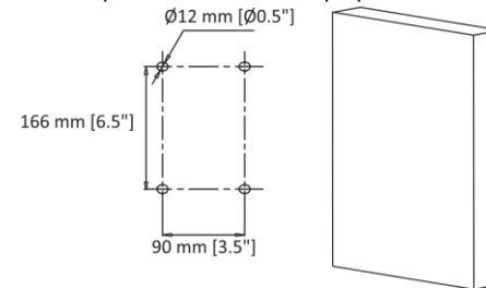
Figura 3-1 Găuriți perețele
