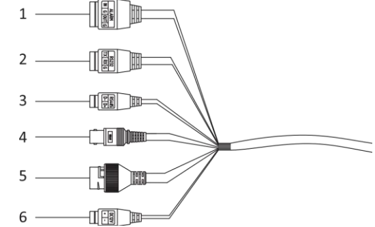
Şekil 2-2 Kamera Kabloları
