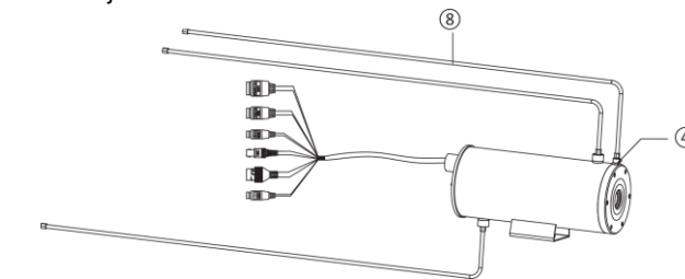
Afbeelding 3-11 Ontstoffingsinstallatie
