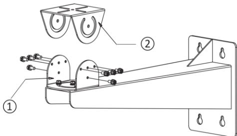
Abbildung 3-3 PT-Gelenk demontieren
