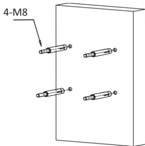
그림 3-1 벽면 드릴 구멍
