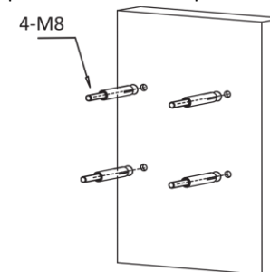
Рисунок 3-2. Укрупіть гвинти M8 в отвори
