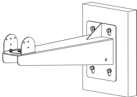
Рисунок 3-4. Установка кронштейна
