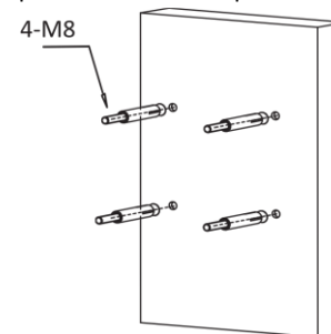
Рисунок 3-2. Установка винтов M8 в отверстия
