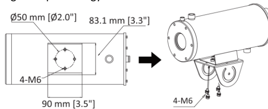
3-6 ábra Rögzítse a páasztázó-billenő csukló felső részét a kamerára
