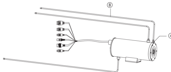
Abbildung 3-11 Entstaubende Installation
