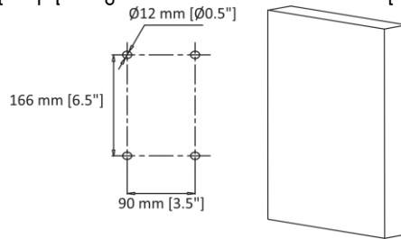
ပုံ 3-1 နံရံပေါ်တွင် အပေါက်များဖောက်ပါ။
