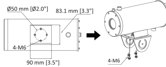
Şekil 3-6 PT Bağlantısının Üst Kısmını Kamerayla Birlikte Takın
