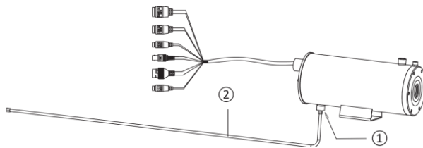
Afbeelding 3-8 Buisaansluiting voor luchtkoeling
