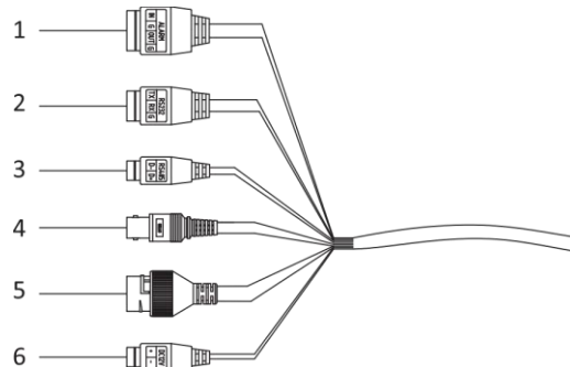
Obrázok 2-2 Káble kamery
