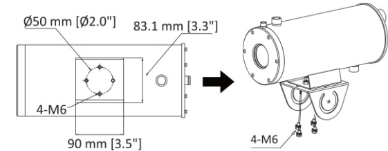
Gambar 3-6 Pasang Bagian Atas Sambungan PT dengan Kamera
