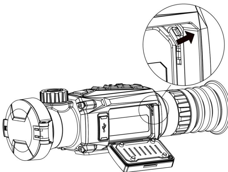
Figura 2-3 Quitar el pestillo de la pila
