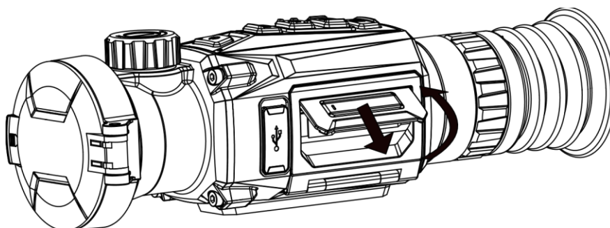
Figura 2-2 Retirar la tapa del compartimiento para las pilas
