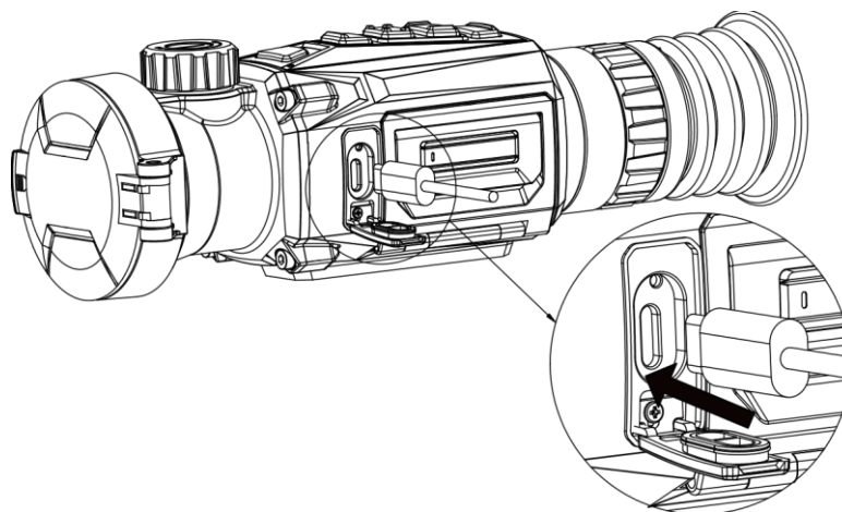
Figura 2-1 Conexión del cable
