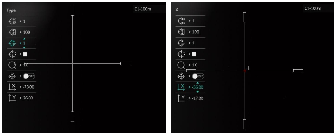
Figura 2-9 Puesta a cero
