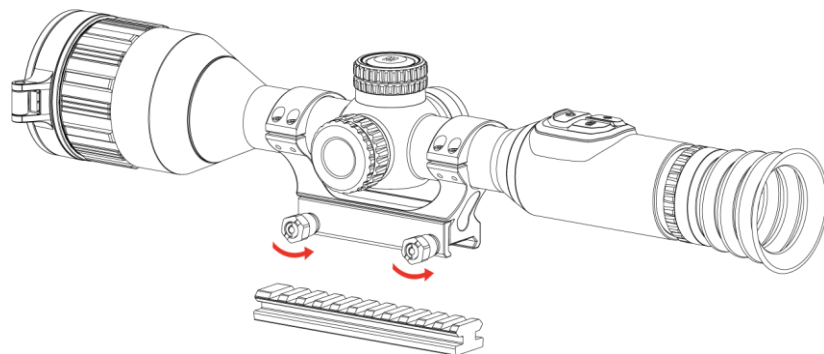
Figur 2-8 Løsne skruene
