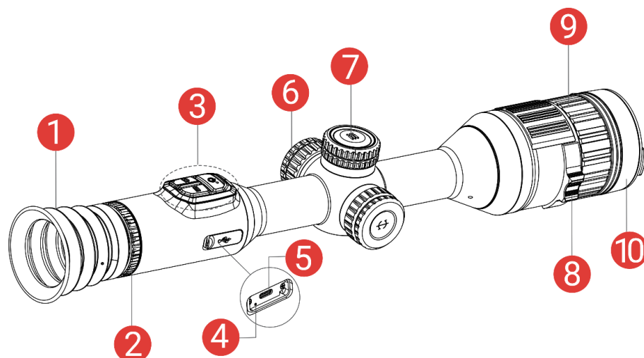
Figura 1-1 Aspetto
