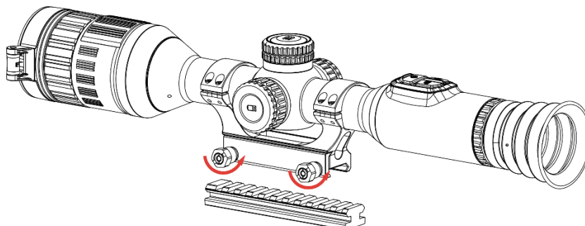
Figura 2-8 Allentamento delle viti
