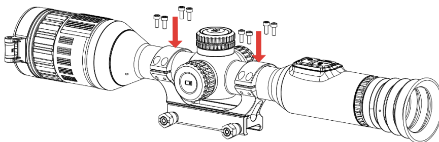
Figura 2-7 Serraggio delle viti
