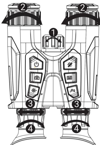
Figur 3-1 Juster enheten
