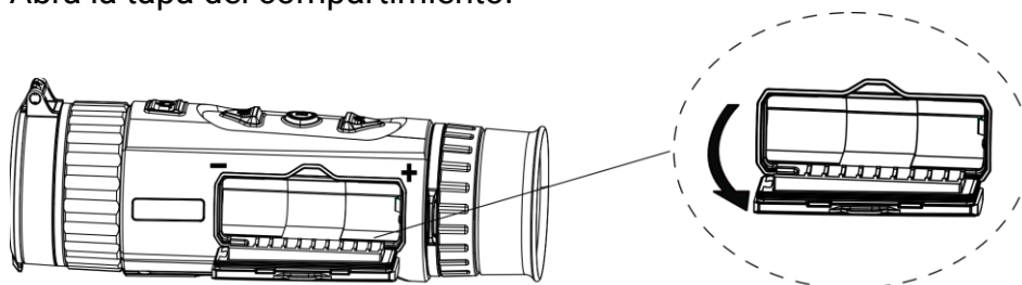
Figura 2-2 Abrir la tapa del compartimiento de la batería
