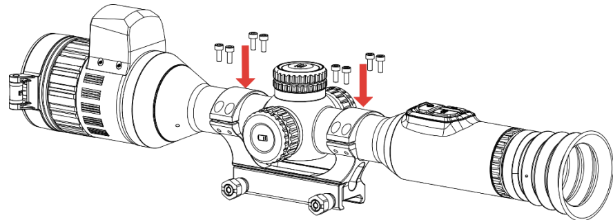
Figura 2-7 Apretar los tornillos
