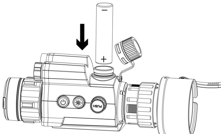
Obrázok 2-4 Inštalácia batérie
