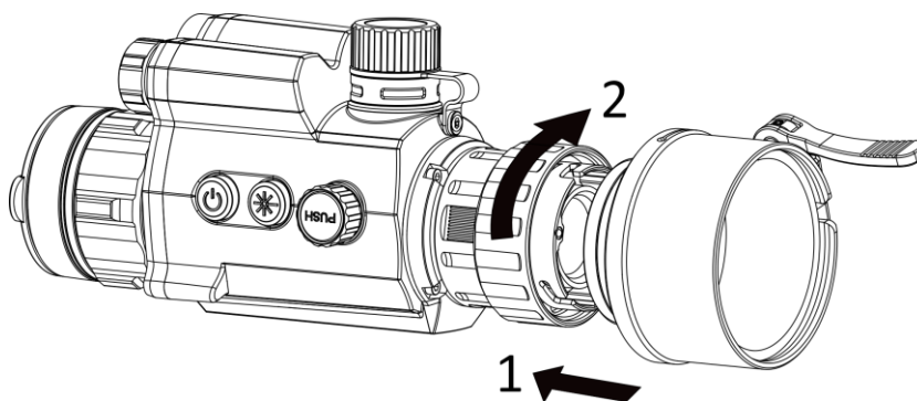
Obrázok 2-2 Inštalácia adaptéra
